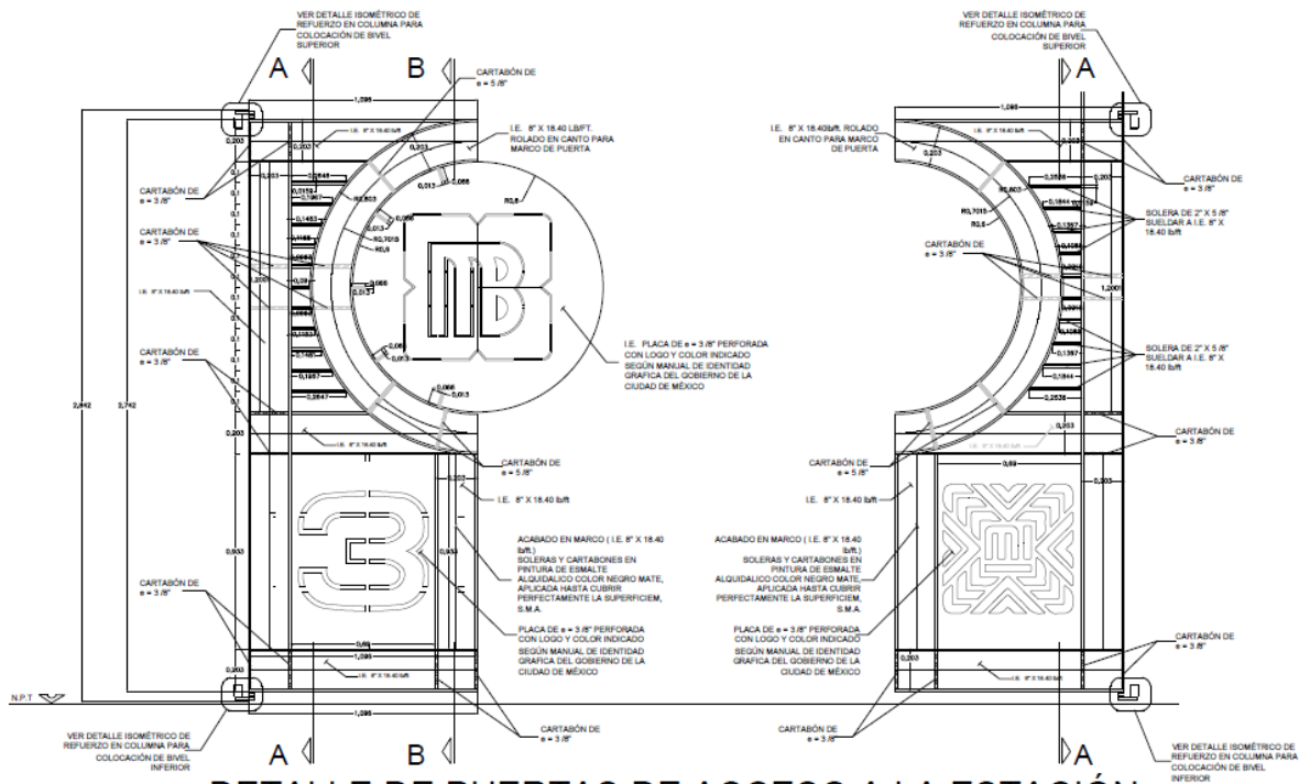
DETALLE DE PUERTAS DE ACCESO A LA ESTACIÓN
