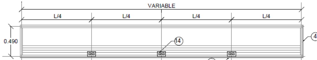
PLANTA DE BASTIDOR DE CAJA METÁLICA
