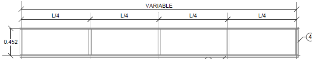
ALZADO DE BASTIDOR DE CAJA METÁLICA
