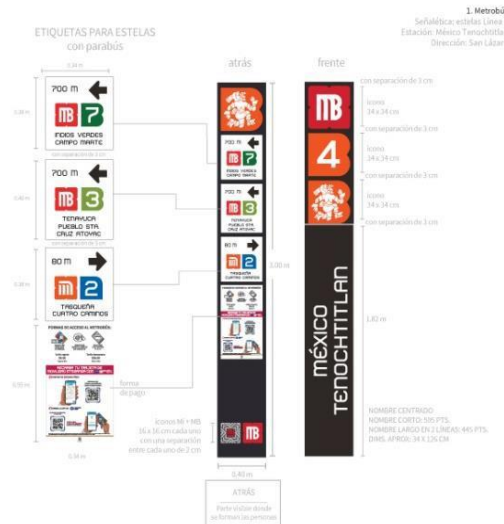
Diseño de estela 2 (con parabús)
